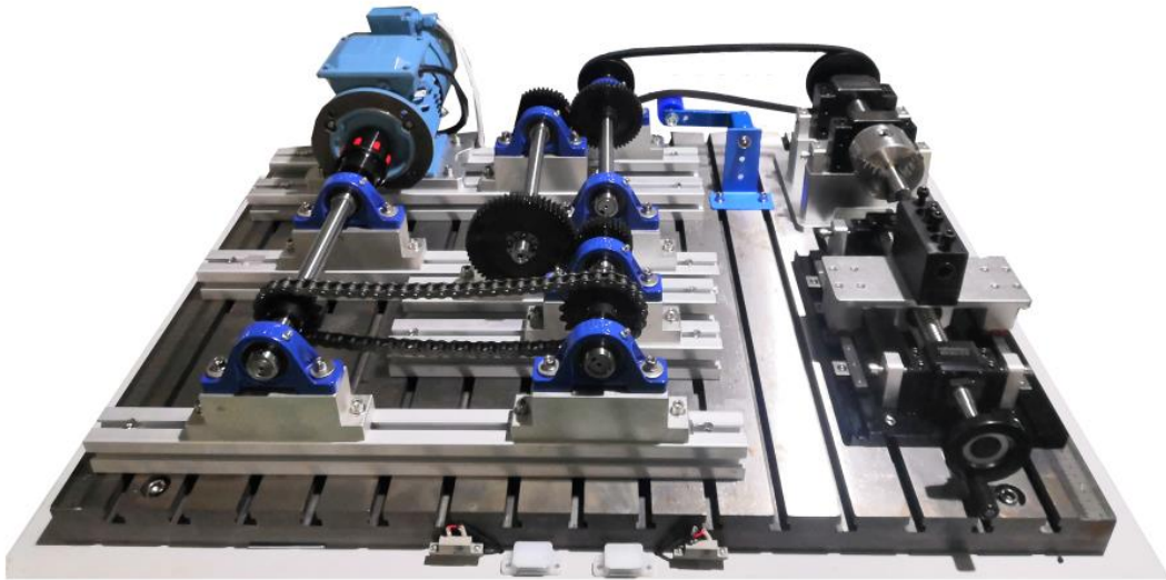
图 4 YTLGC-5A 型工业机械传动竞赛平台台面
