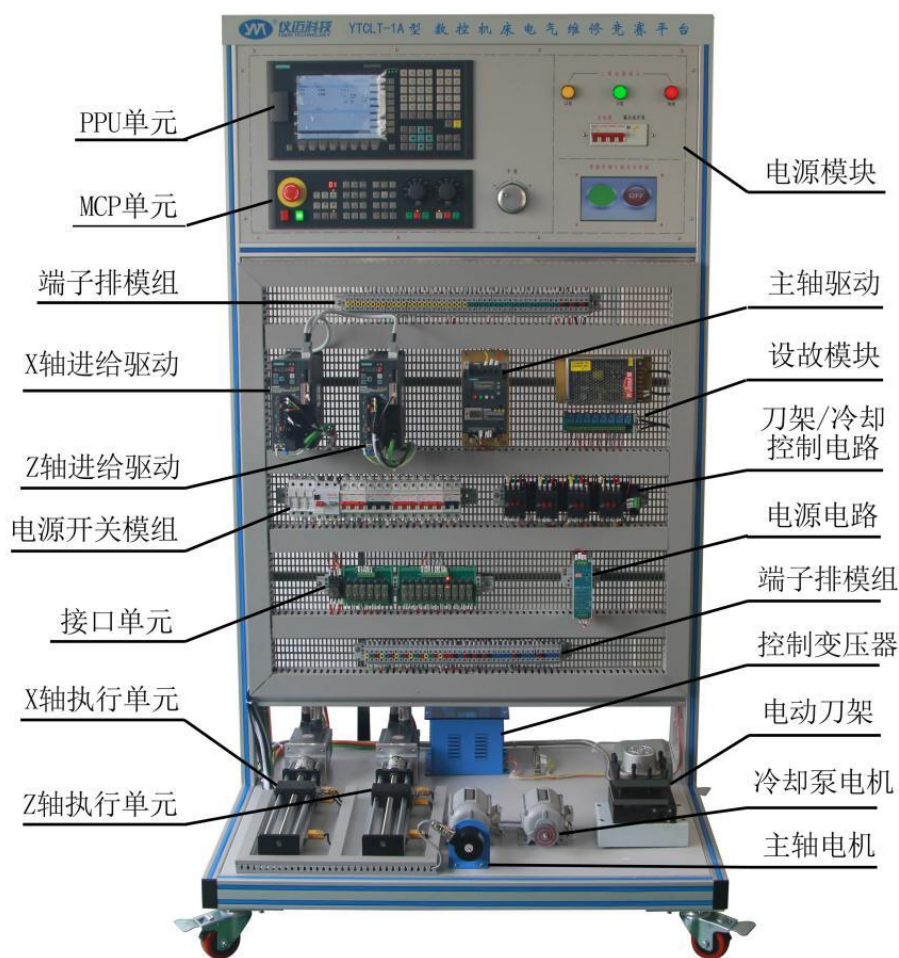
图 2 YTCLT-1A 型数控机床电气功能测试与排故竞赛平台
